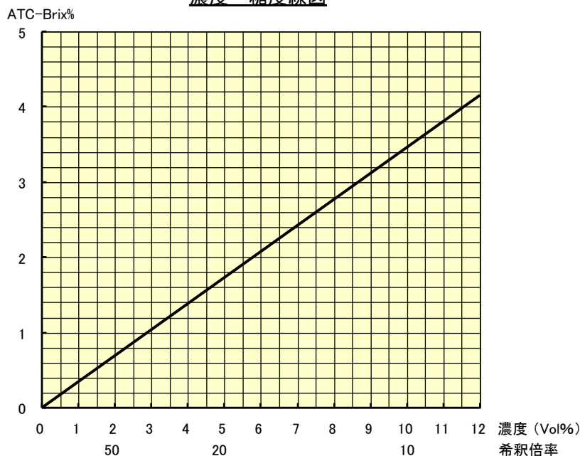
濃度—糖度線図
